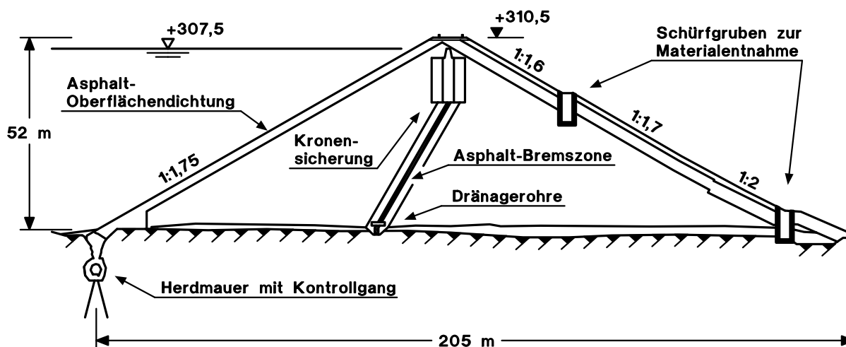
Bild 1: Querschnitt des Biggedamms mit Lage der Schürfguben
